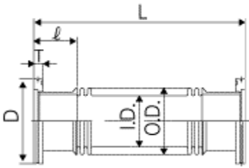
ISO-MF 플렌지 타입 일람 <단위: mm>
