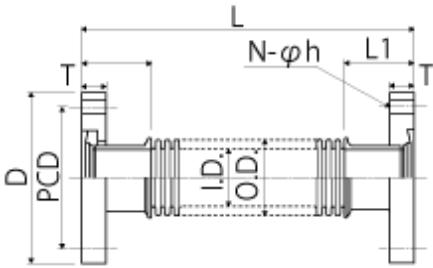
CF 플렌지타입 일람 <단위: mm>
