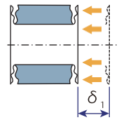
\delta_1 : 축방향변위량
