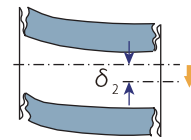
\delta_2 : 축직각방향변위량
